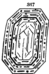
Angite.
